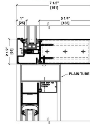
5 1/4" HORIZONTAL TUBE/SERIES 175 DOOR
