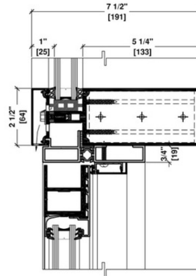
5 1/4" HORIZONTAL TUBE/SERIES 260 DOOR
