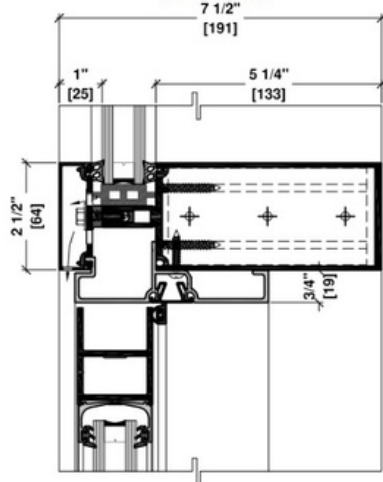
5 1/4" HORIZONTAL TUBE/SERIES 175 DOOR
