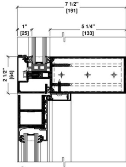
5 1/4" HORIZONTAL TUBE/SERIES 260 DOOR
